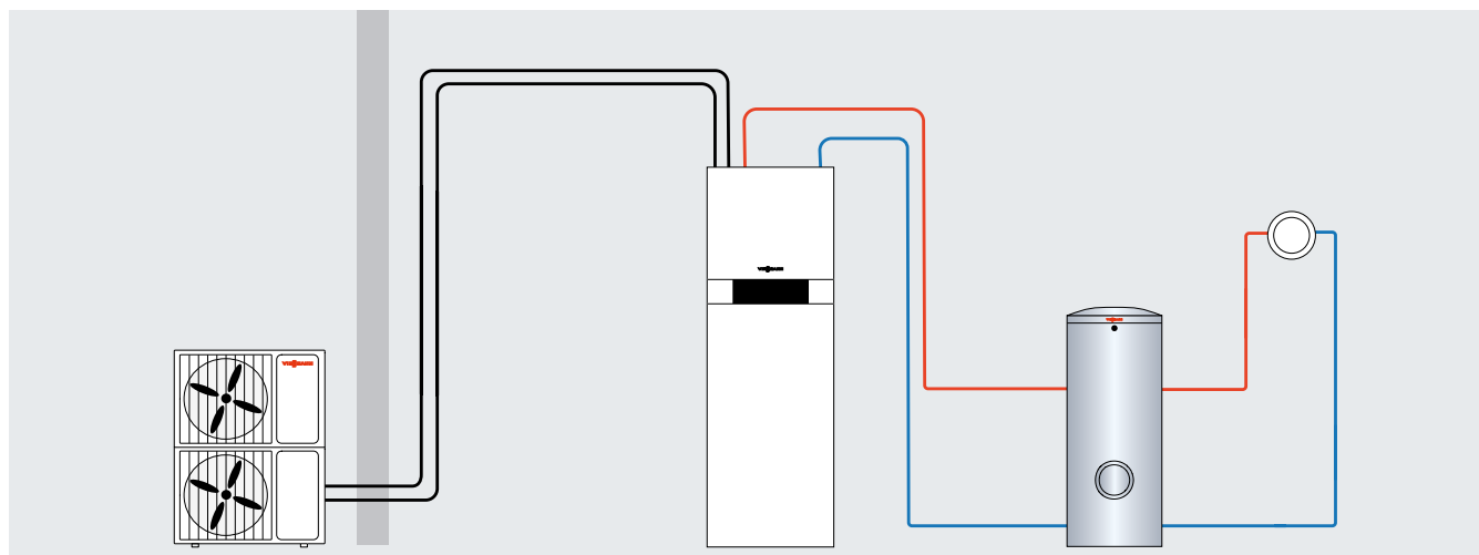
Vitocal 111-S: schema di applicazione
